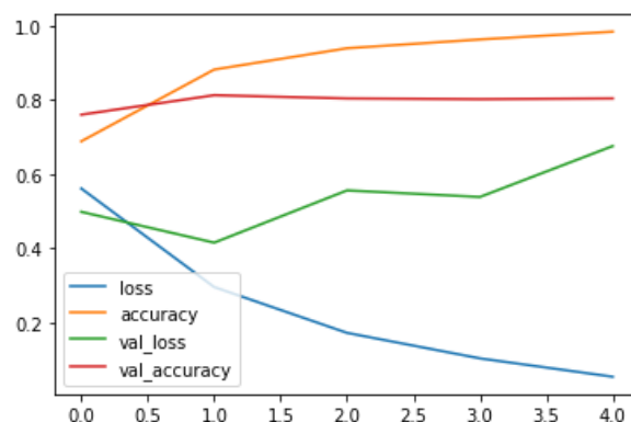
GRU
